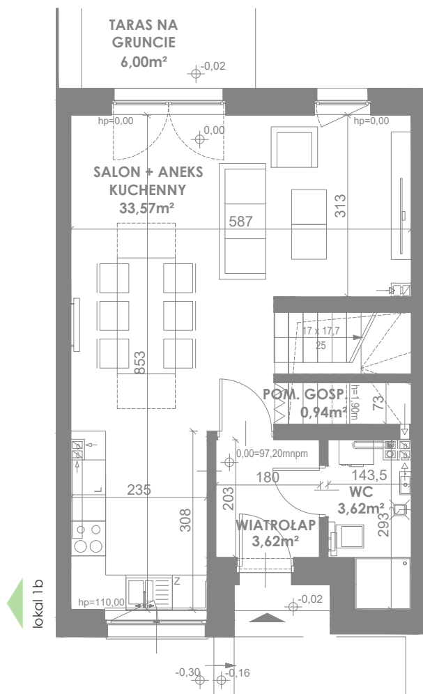
RZUT PARTERU
