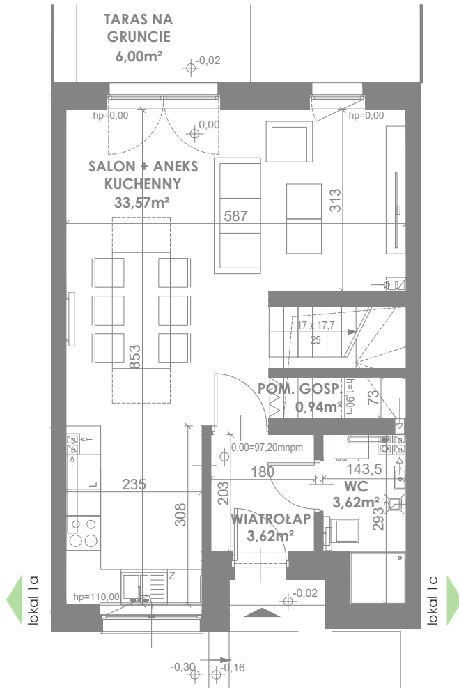
RZUT PARTERU
