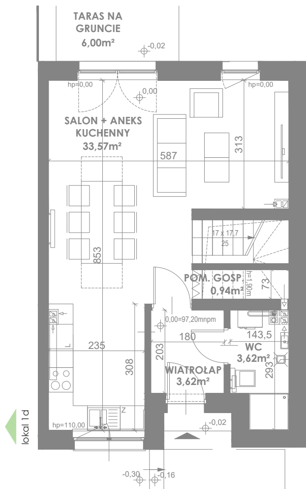
RZUT PARTERU
