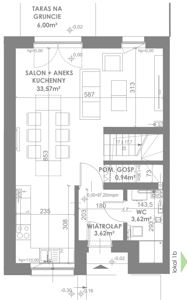
RZUT PARTERU
